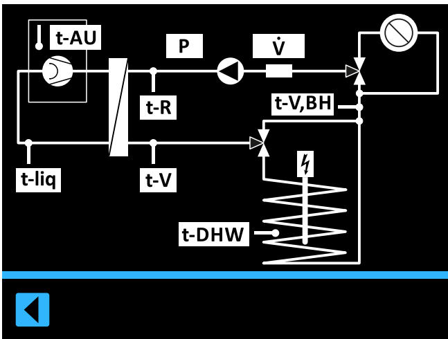
Bild 4-7 Hydraulikscharbild - Erste Seite
