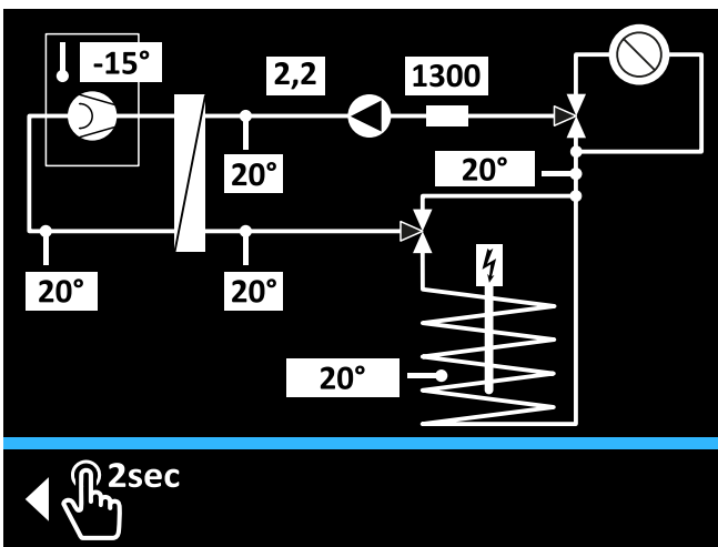
Bild 4-8 Hydraulikscharbild - Zweite Seite
