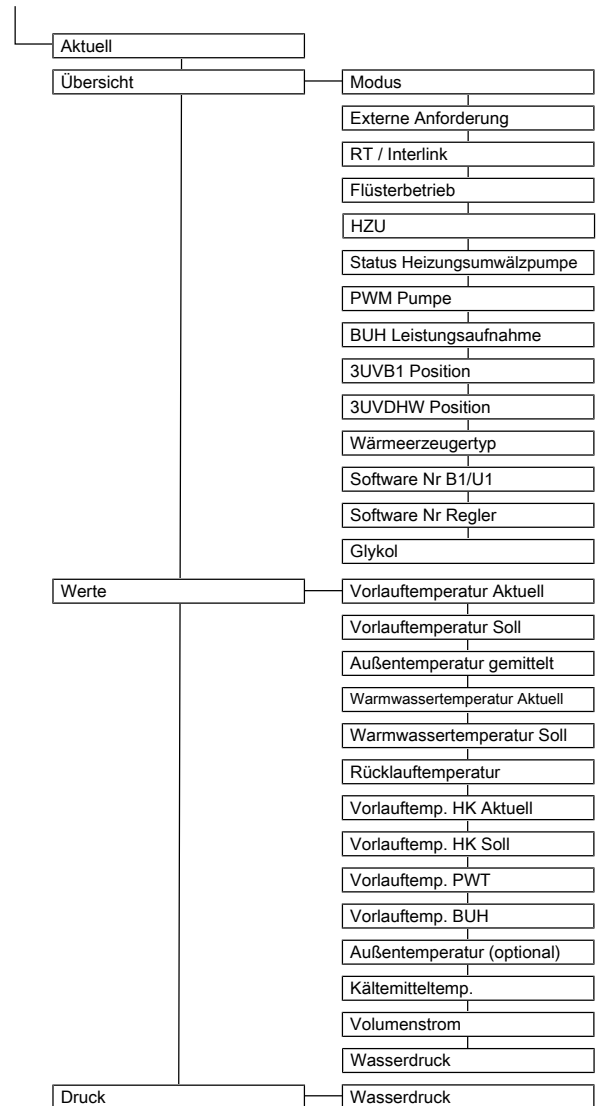
Bild 6-6 Parameter im Menü: "Info"
