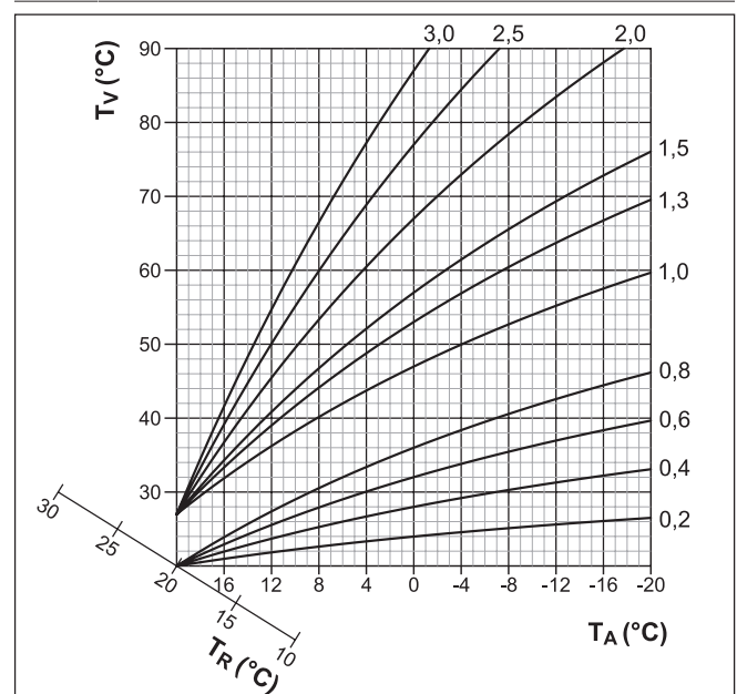
Bild 4-2 Heizkurven T_A Außentemperatur T_R Raumtemperatur-Sollwert T_v Vorlauftemperatur
