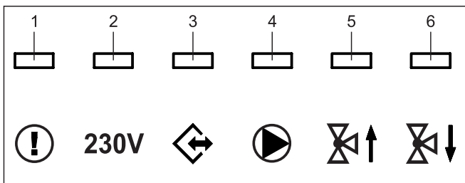
Bild 9-2 Symbolerklärung Statusanzeigen EHS157068
